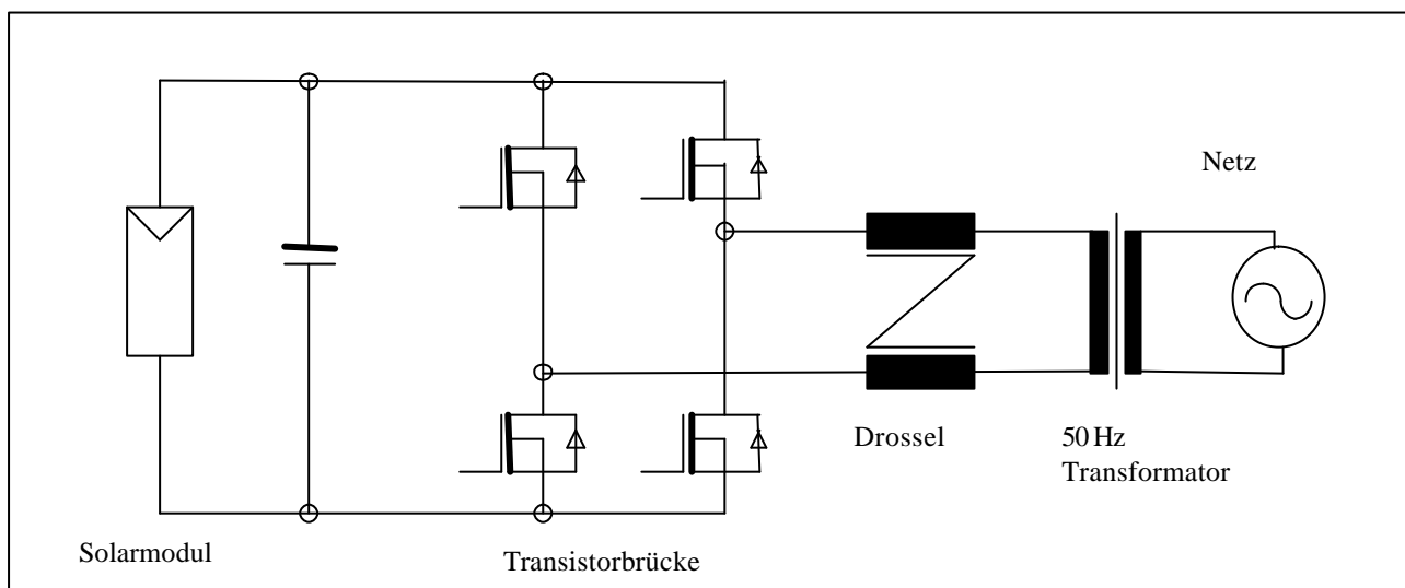
Abb. 1: Modulwechselrichter mit NF-Ringkerntransformator
